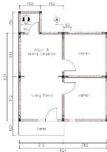
DENAH RUMAH RUSPIN TYPE 36
