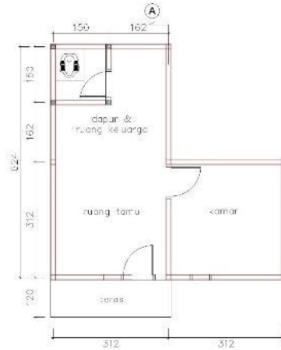
DENAH RUMAH TYPE 36 (inti luas 27)
